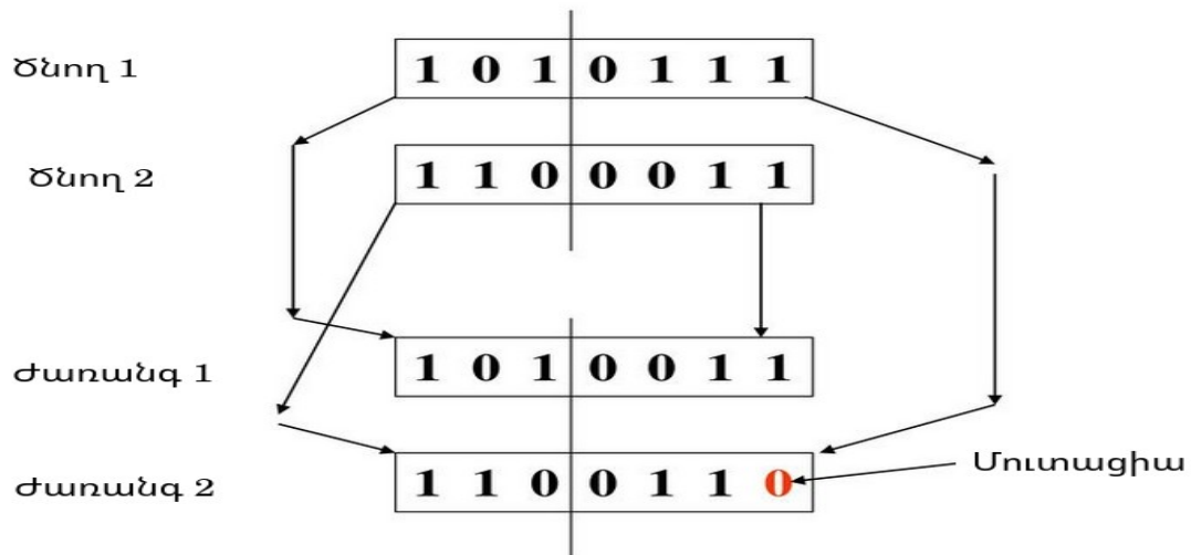
Նկար 2.4 Մուտացիա օպերատորի կիսումը խաչասերման օպերատորից կիրառումից հետո
